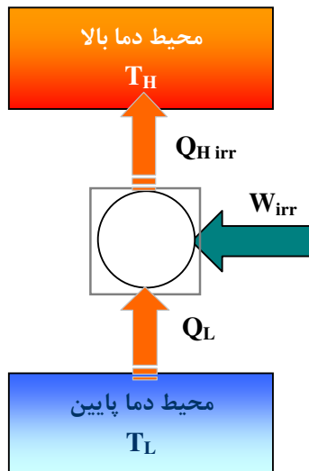
شکل ۵-۲۴. پمپ حرارتی برگشت‌ناپذیر
